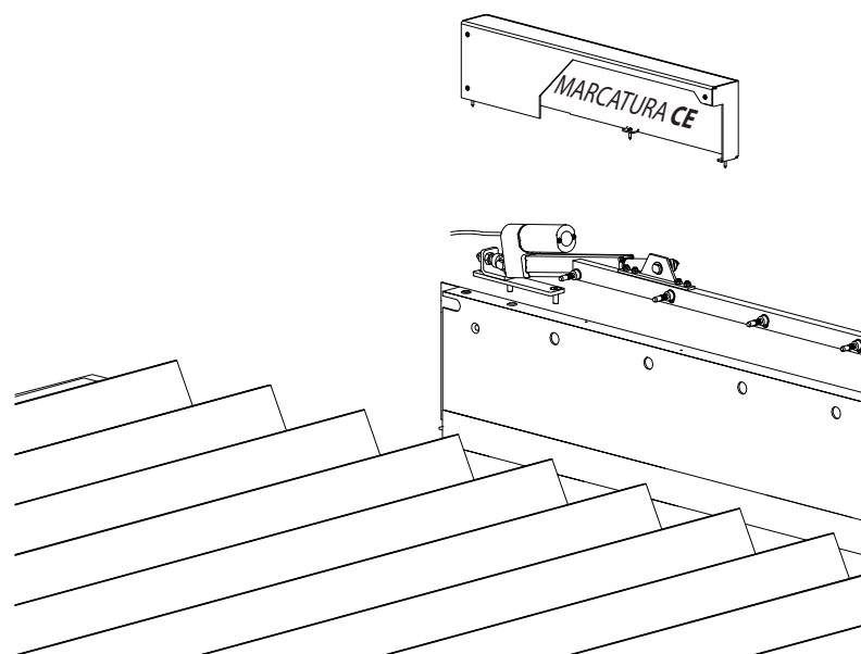
Posizione sulla struttura dell'etichetta con la marcatura CE
