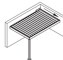
Situación constructiva 3 Pared // Span y Pared // Pivot
